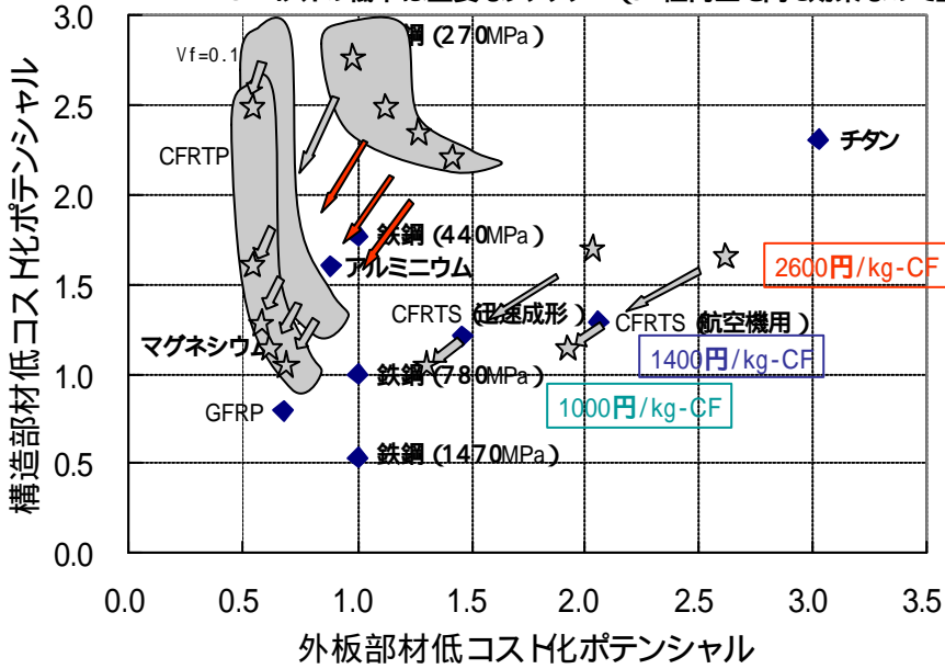
図 A4 各種軽量素材による外板部材と強度部材の低コスト化ポテンシャル 数値は鉄鋼 (780MPa) との比、数値が小さいほど低コスト化できる CFコストの低下は重要なファクター (3R性向上も同じ効果なので重要)
