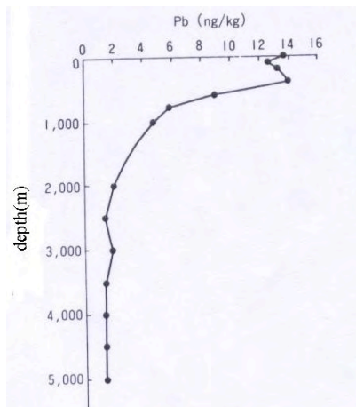
中部北大西洋の鉛濃度
