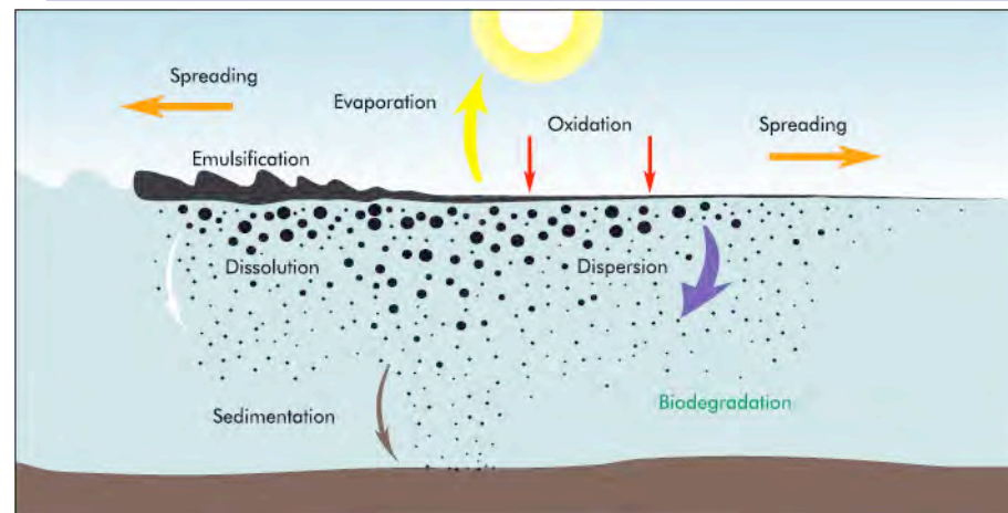
流出油の挙動
