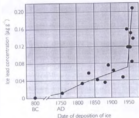
グリーンランドの氷中の鉛濃度
